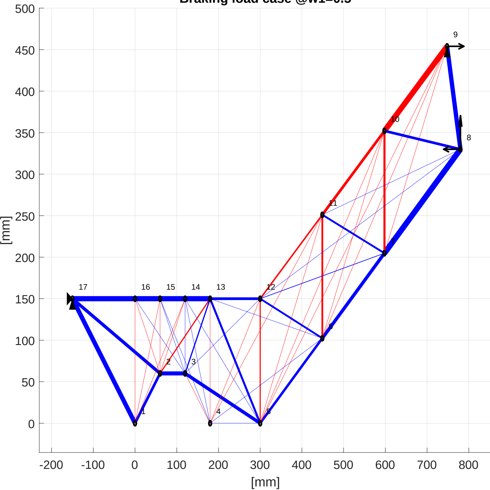
Braking load case @w1=0.5
